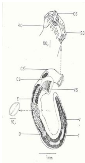
Echinostoma sp
