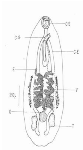
Paramonostomum alveatum
